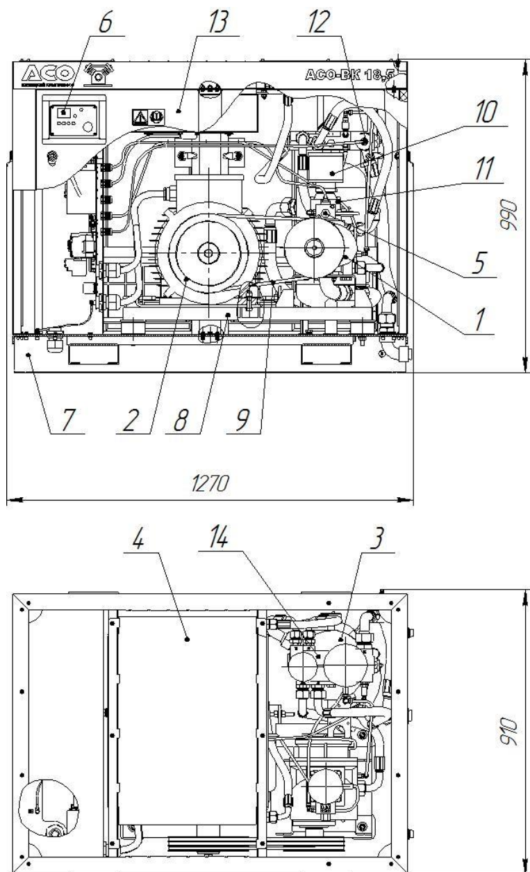
Рисунок 2. Агрегат компрессорный.
